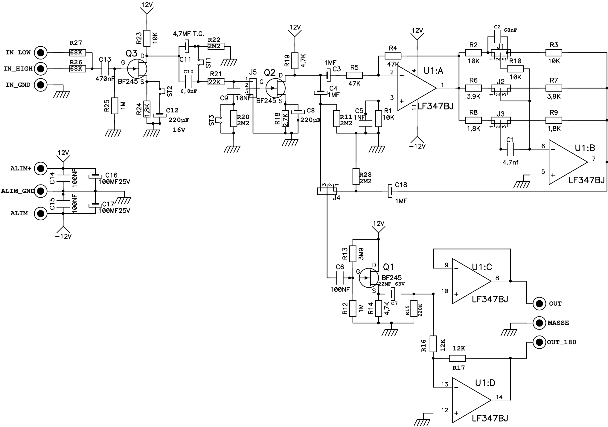
Pre-Ampli GUITARE
