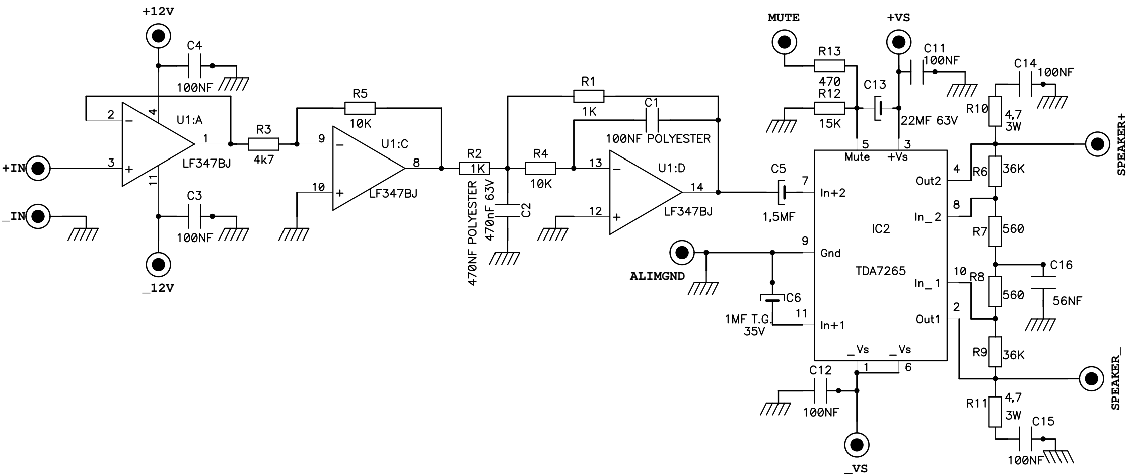
SUBWOOFER version2
